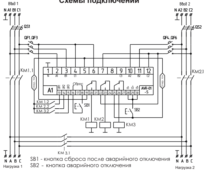
Схема подключения AVR-01-S с контакторами.
